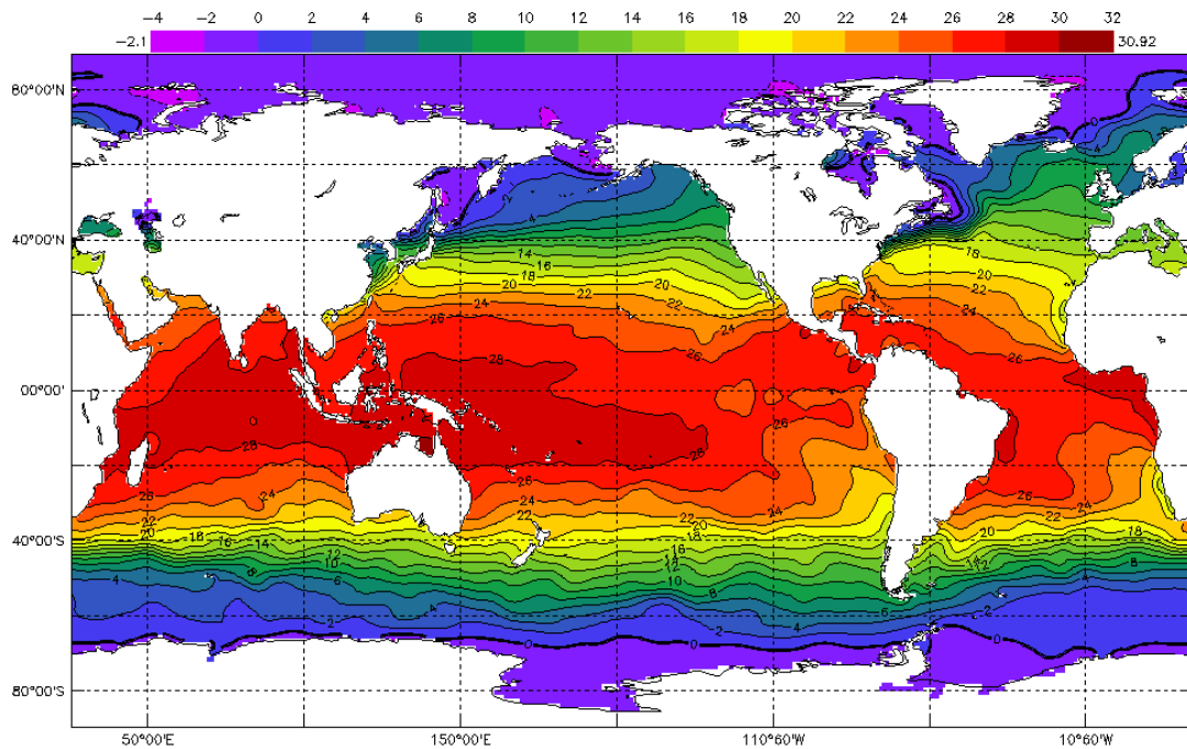
SST_Jan/Feb2011
